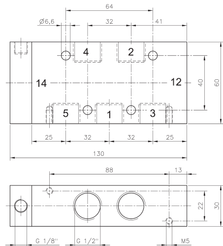
P 510 121 G/P 511 121 G
